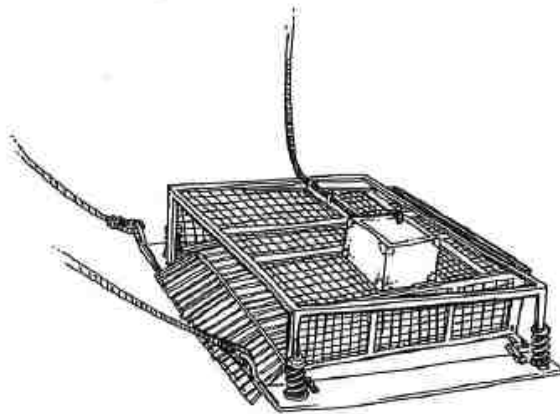
Figura 19. Vibrantino (fonte: Provincia di Venezia, 2011).
