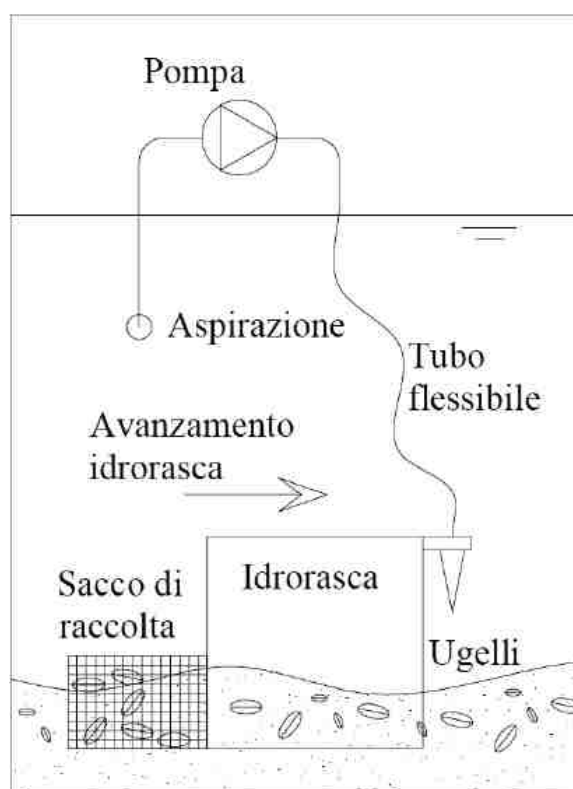
Figura 30. Schema idraulico di funzionamento di una idrorasca con relativa motopompa associata (fonte: Provincia di Ferrara, 2007).
