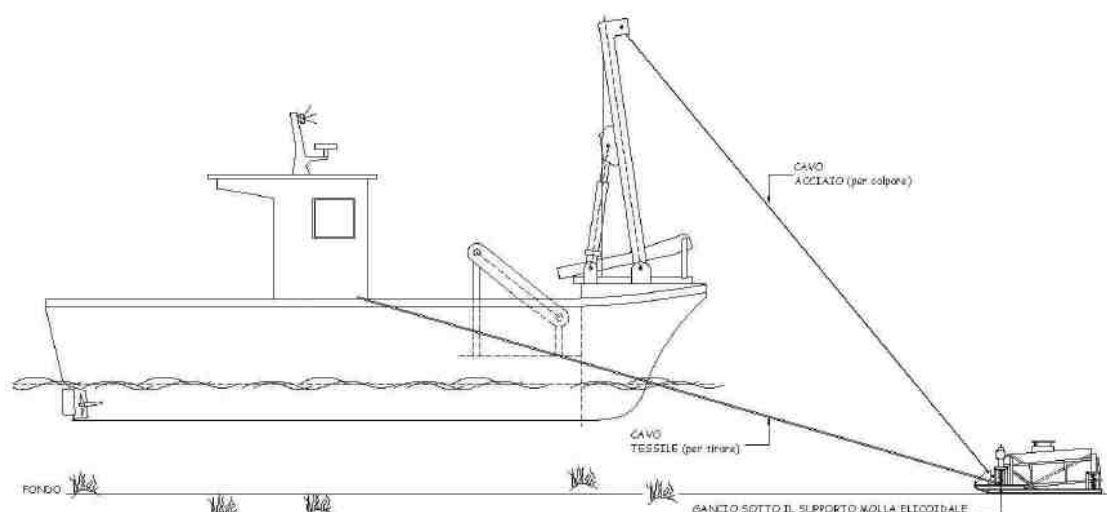
Figura 22. Vibrantino, visione d'insieme (fonte: Consorzio Mediterraneo S.c.a.r.l. e C.I.R.S.PE, 2003).
