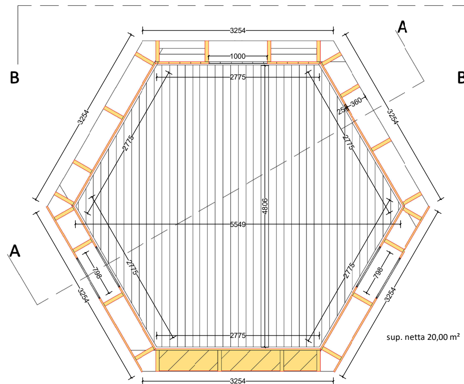
Pianta
