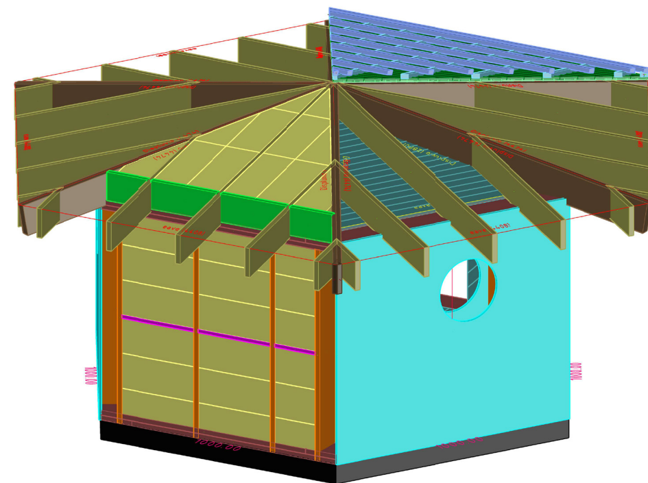
Spaccato 3D
