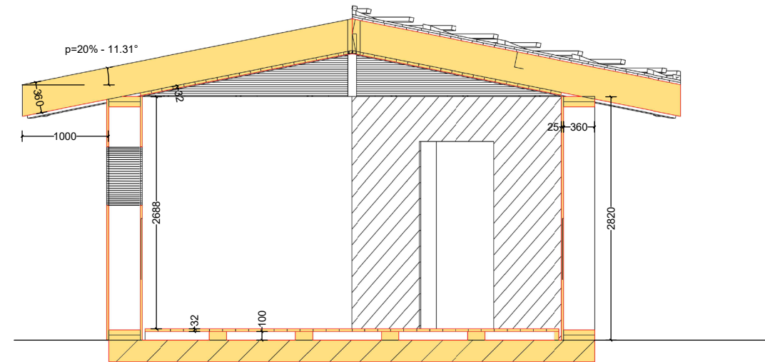
Sez. A-A
